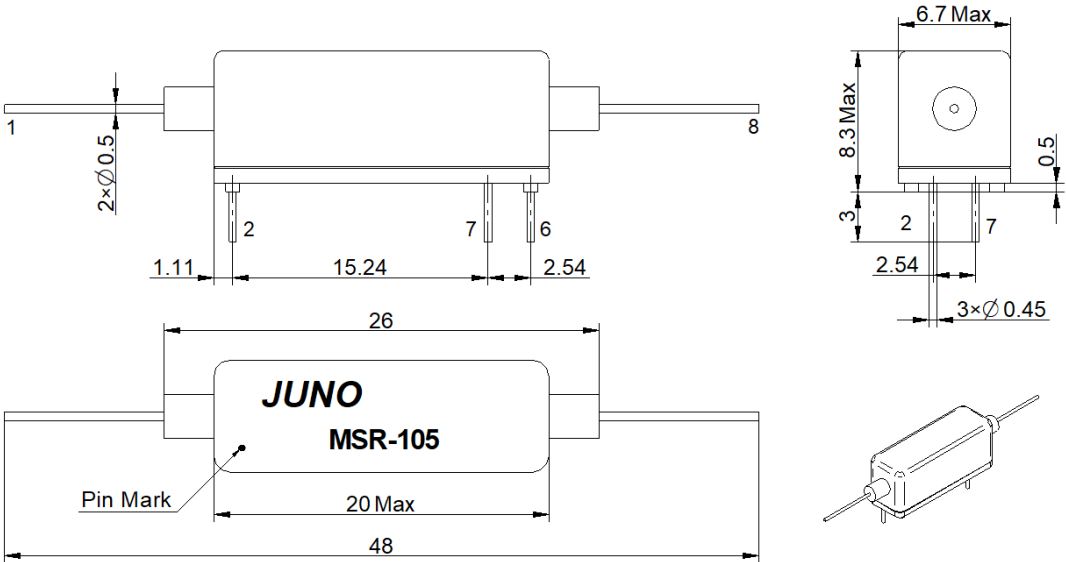
外形图 Outline Dimension
