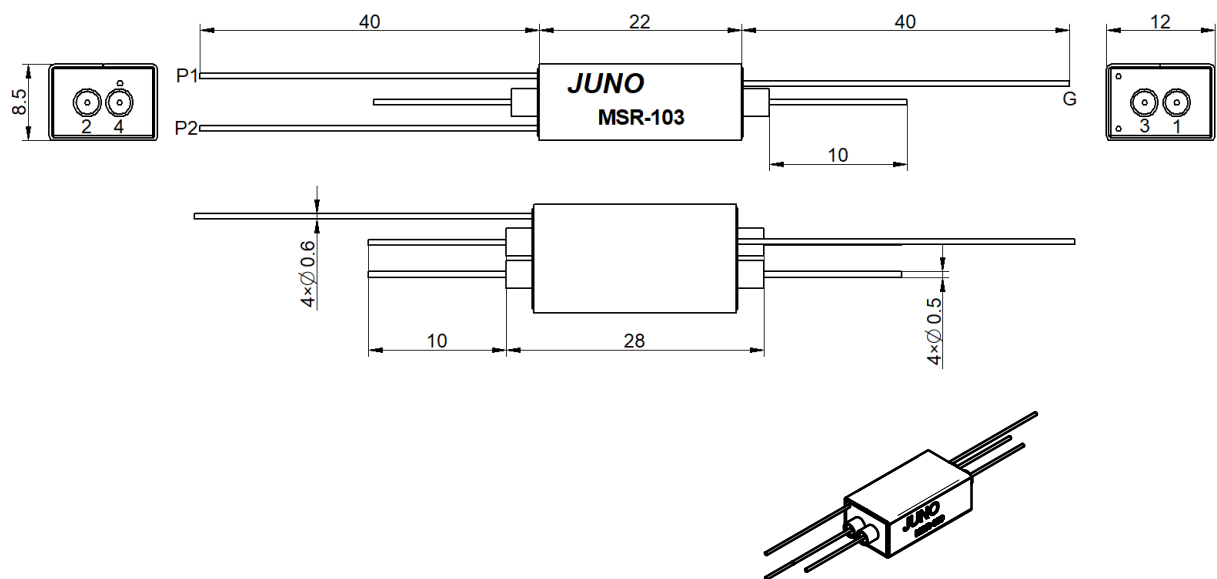
脚位布局图 Pin Layout
