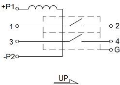
顶视图 Top View
